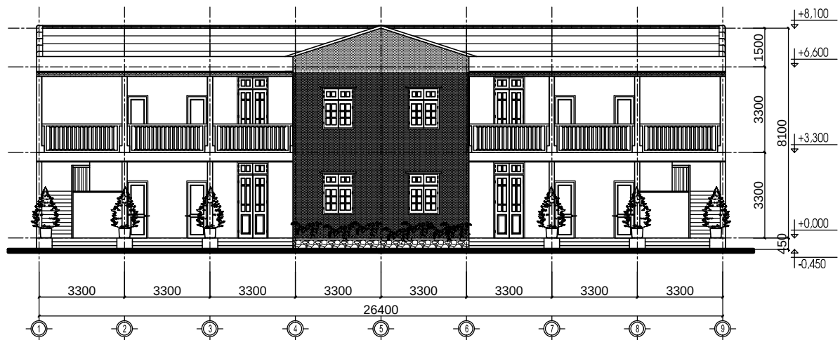
MẶT ĐỨNG TRỰC 1-9
