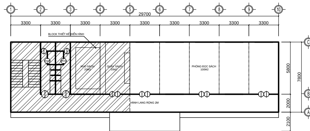
MẶT BẰNG TẦNG 2
