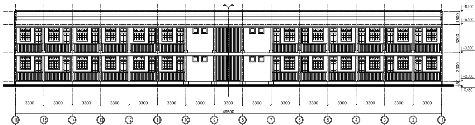
MẶT ĐÚNG TRỰC 16-1
