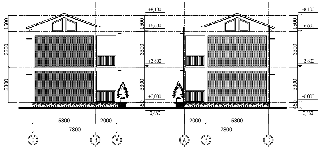
MẶT ĐỨNG TRỰC C-A
