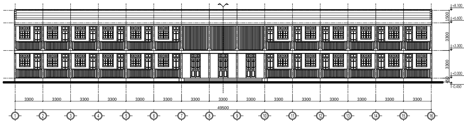
MẶT ĐÚNG TRỰC 1-16
