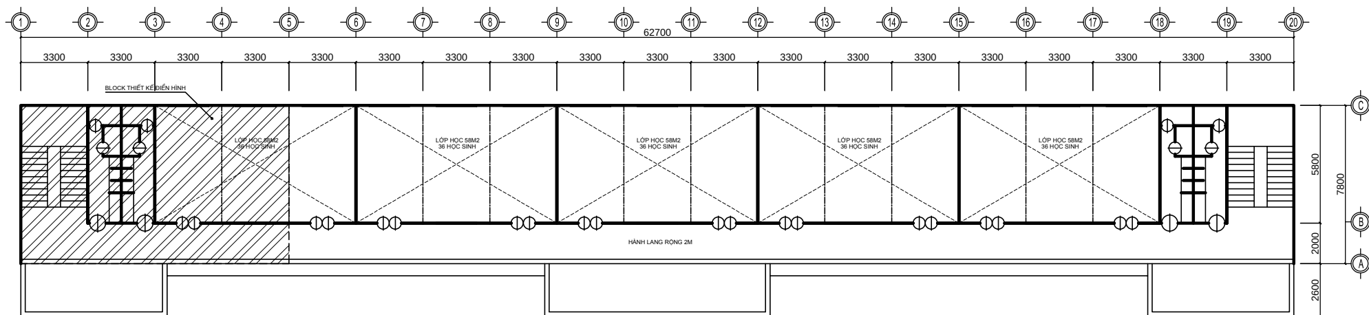
MẶT BẰNG TẦNG 2
