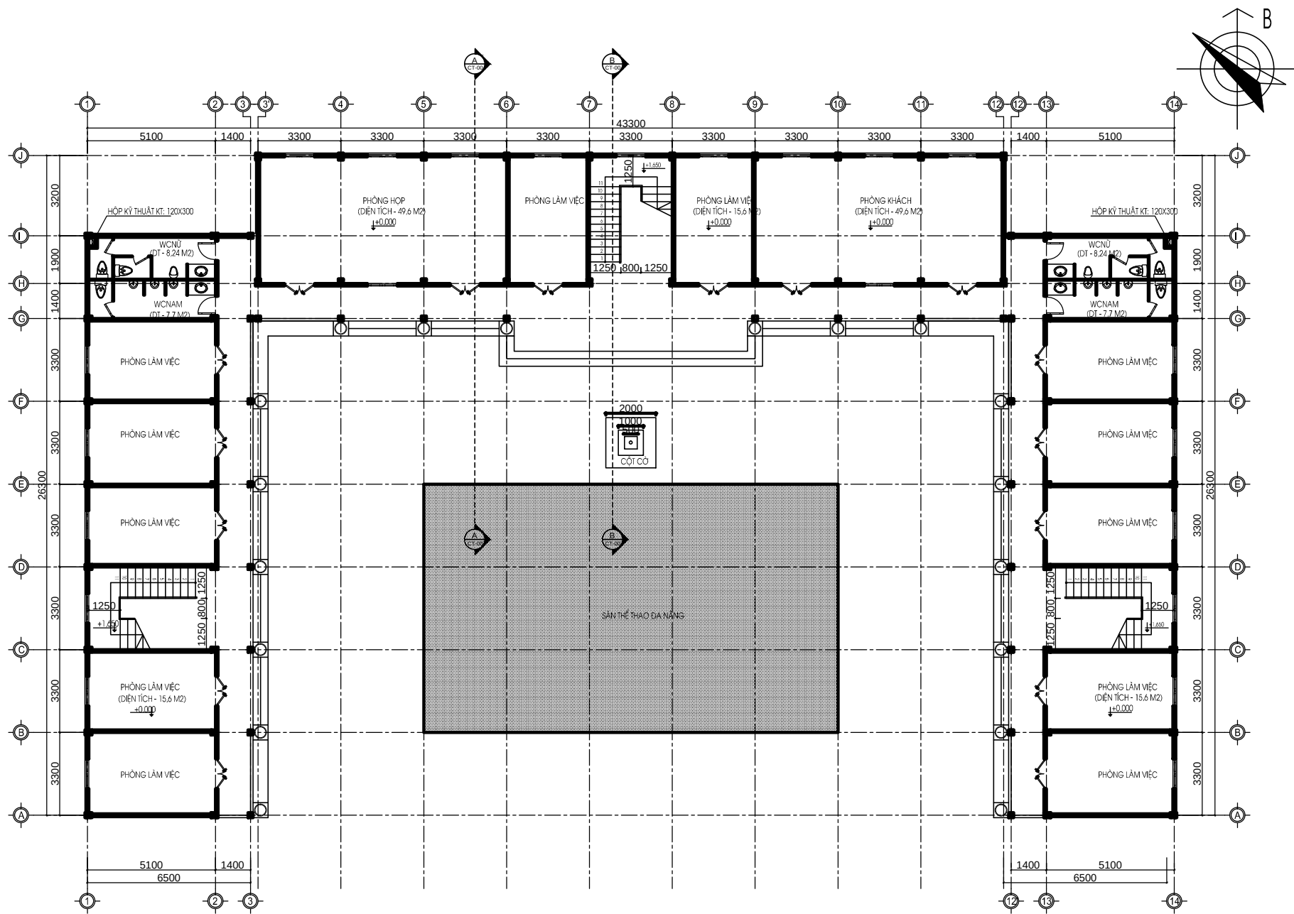
MẶT BẰNG TẦNG 1 TRỤ SỞ LÀM VIỆC
