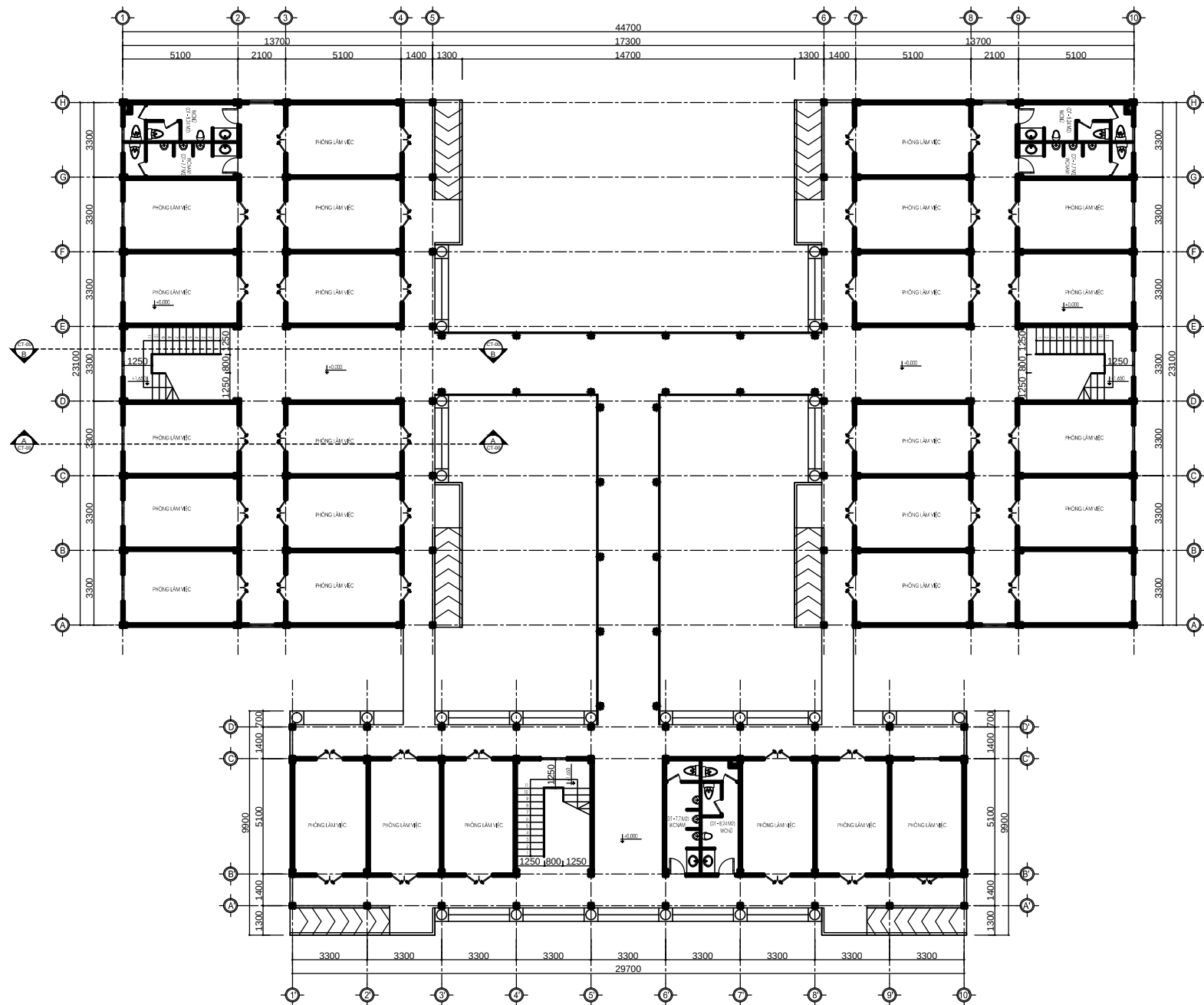
MẶT BẰNG TẦNG 2
