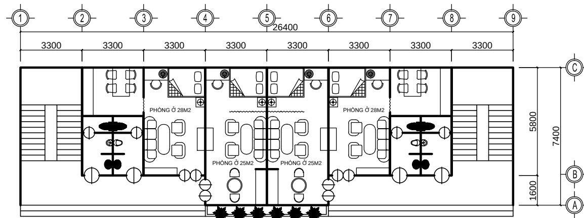
MẶT BẰNG TẦNG 1
