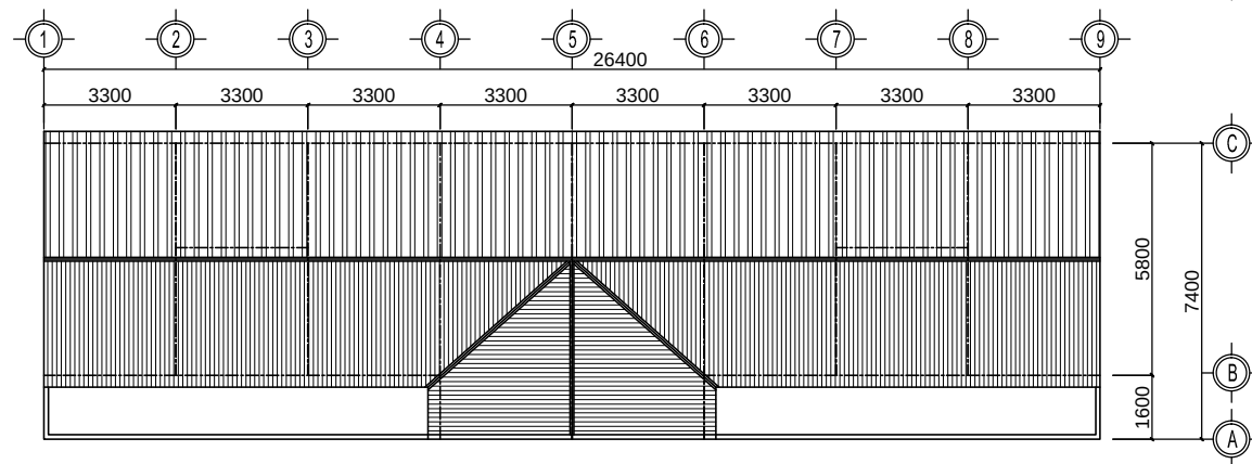
MẶT BẰNG MÁI
