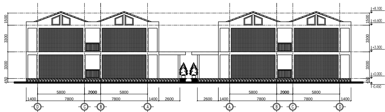
MẶT ĐỨNG TRỤC D-A
